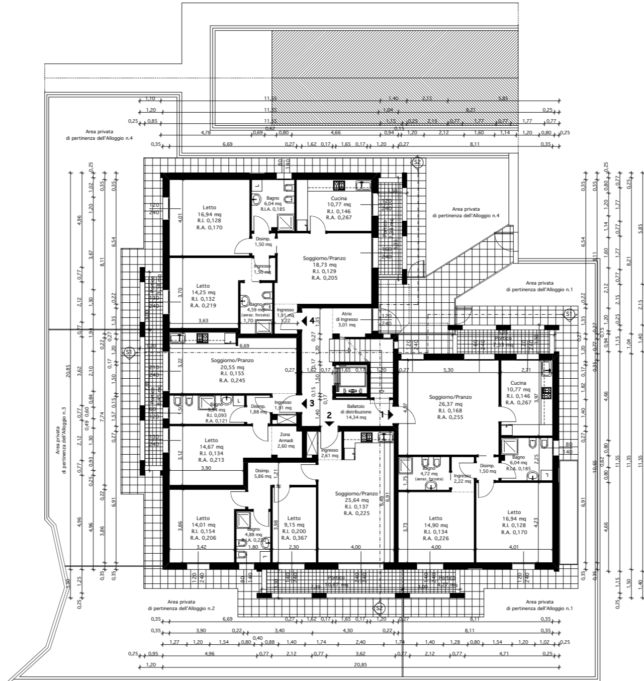
PIANTA DEL PIANO TERRA
